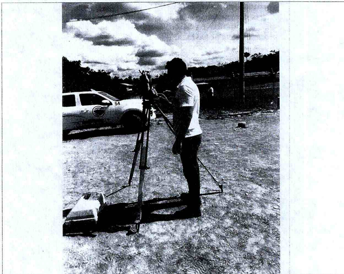
Foto 1: Colocación, Nivelación y ajuste de Estación Total Geomax para Levantamiento Topográfico
