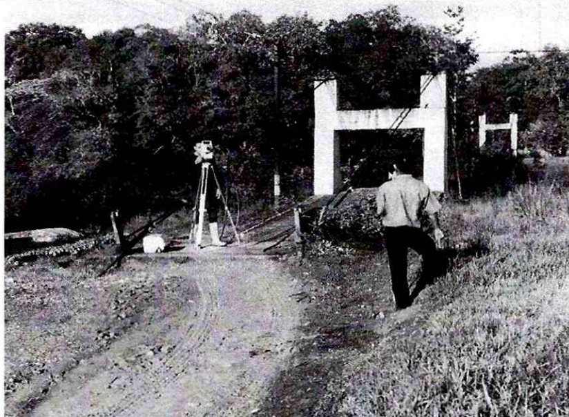
Foto 2: Levantamiento topográfico de laterales y eje de la vía de acceso principal
