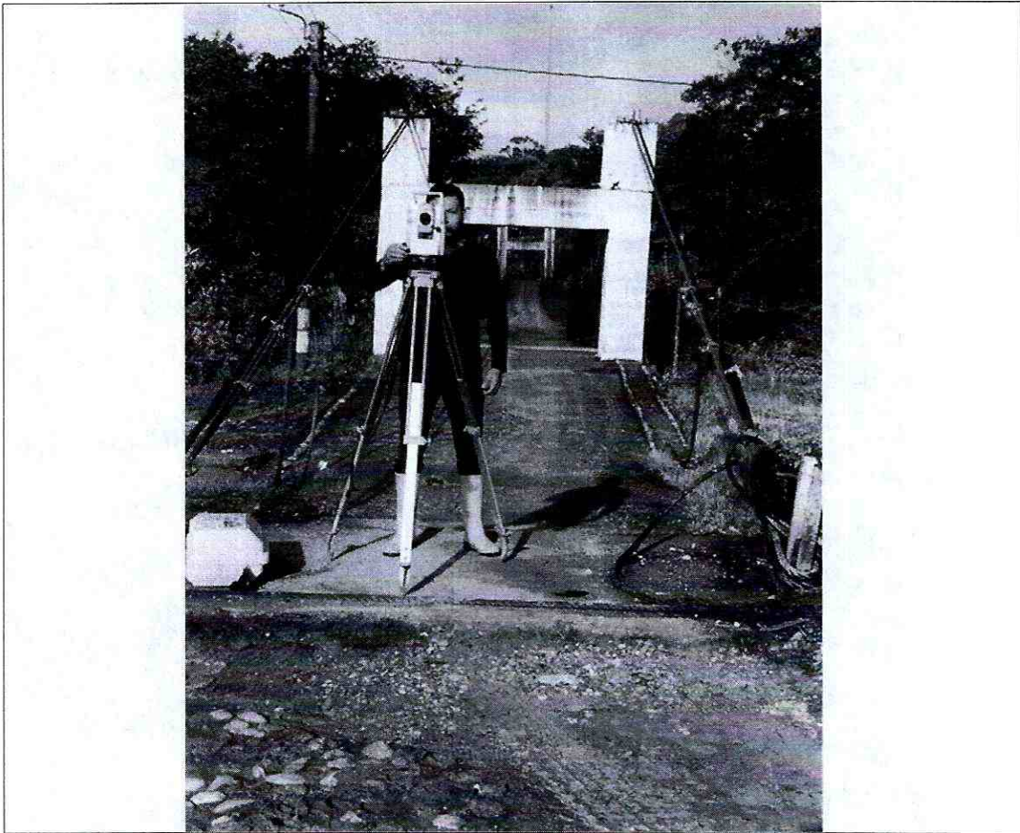
Foto 1: Colocación, Nivelación y Ajuste de Estación Total para Levantamiento Topográfico
