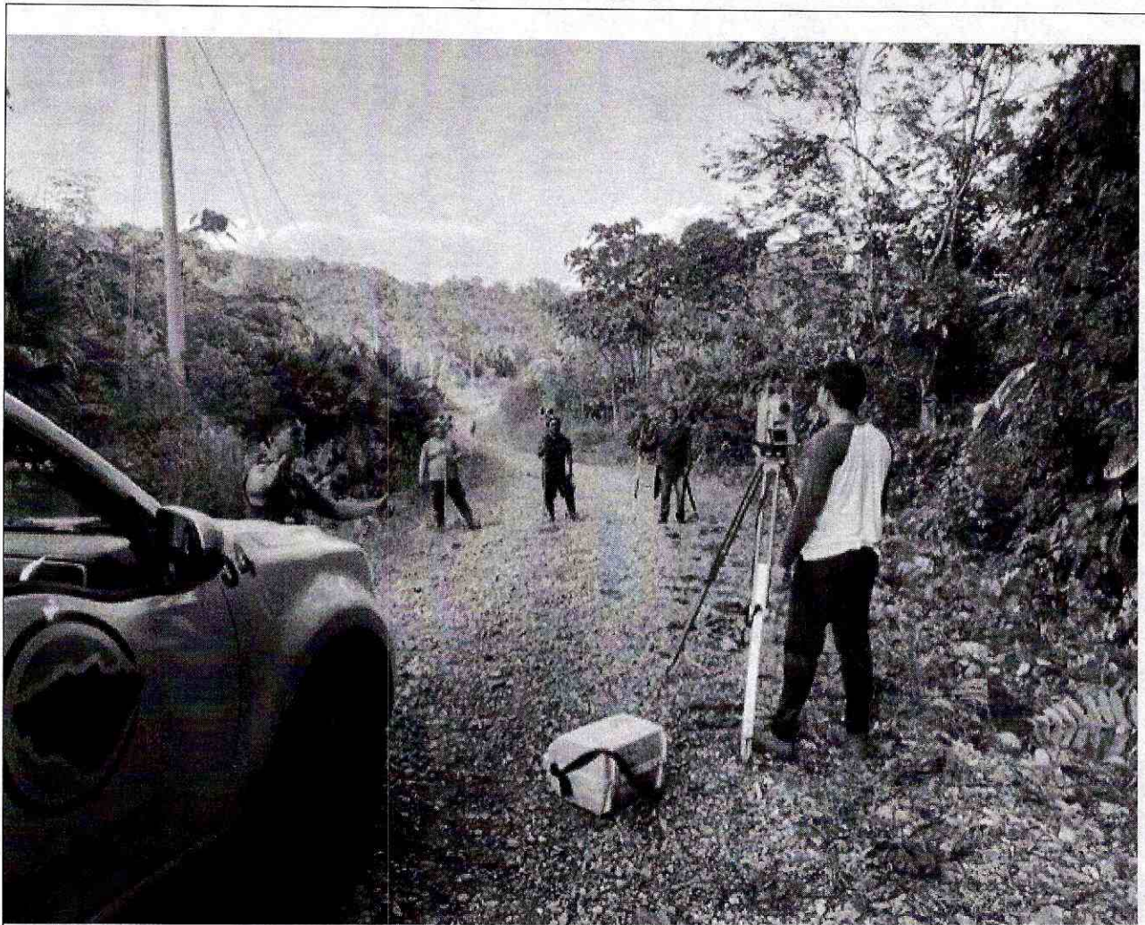
Foto 2: Levantamiento topográfico para proyecto de asfaltado en la Comunidad Meñenpare 1+400
