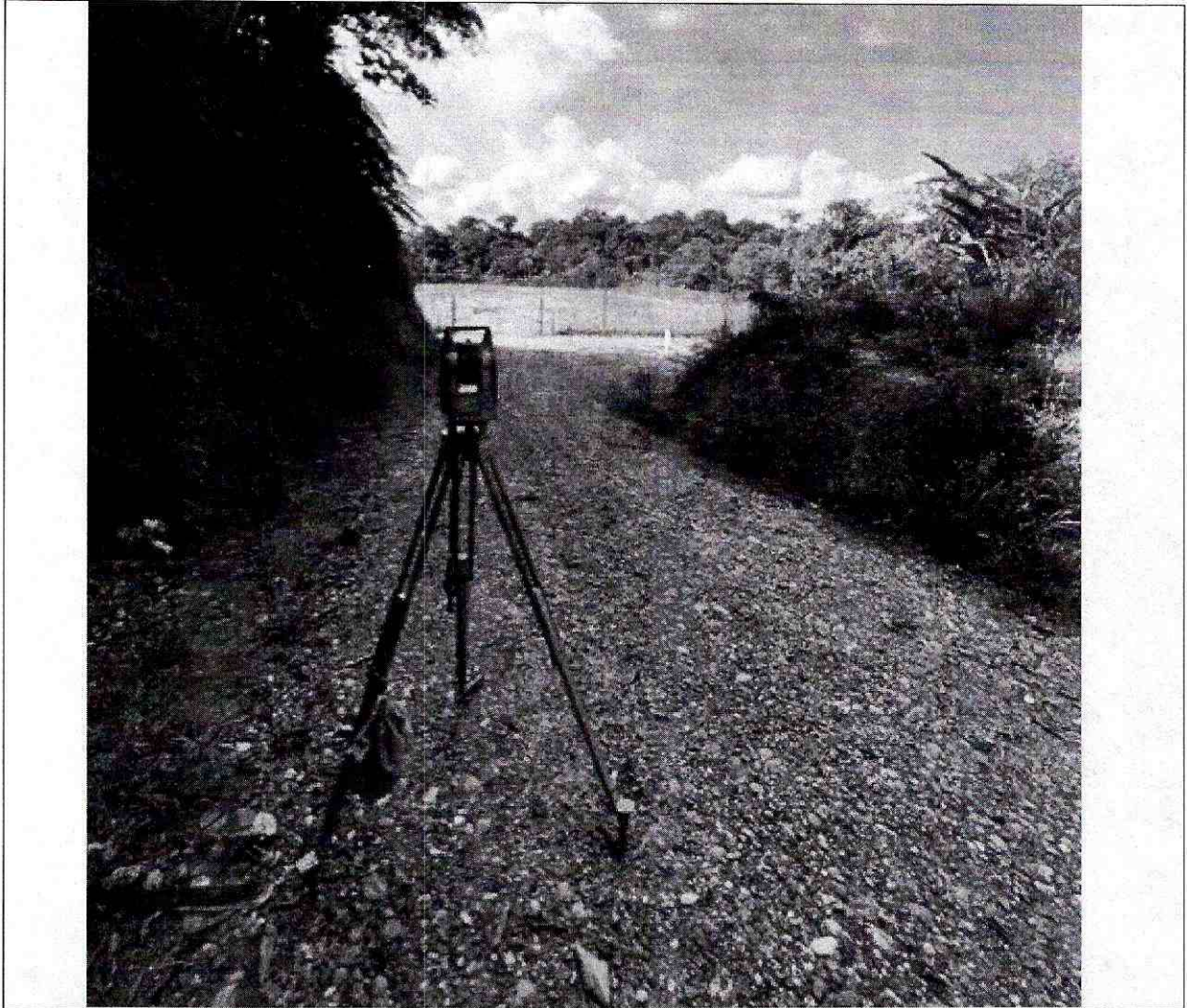
Foto 4: Llegada de levantamiento topográfico del proyecto de asfaltado a la plataforma petrolera abscisa 4+200
