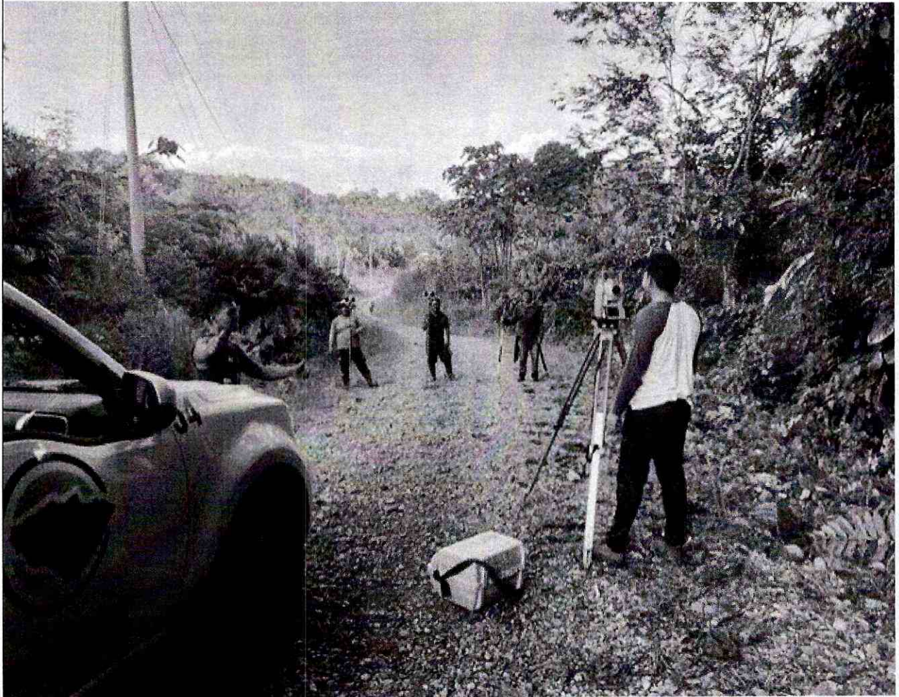
Foto 2: Levantamiento topográfico para proyecto de asfaltado en la Comunidad Meñenpare 1+400
