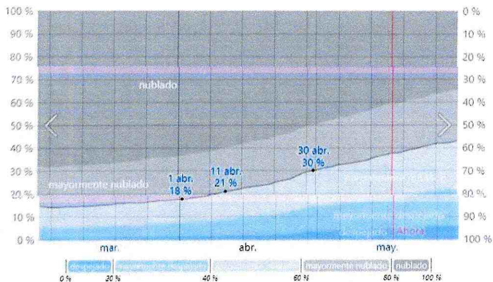
Ilustración 2 Categorías de nubosidad en abril 2023 en Puyo
