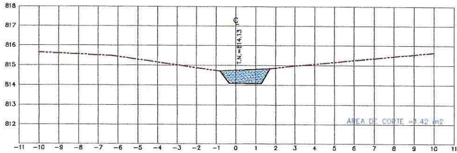
ESTACION 0+193.00 - Lado Izquierdo ESCALA HORIZONTAL 1 : 100 ESCALA VERTICAL 1 : 100
