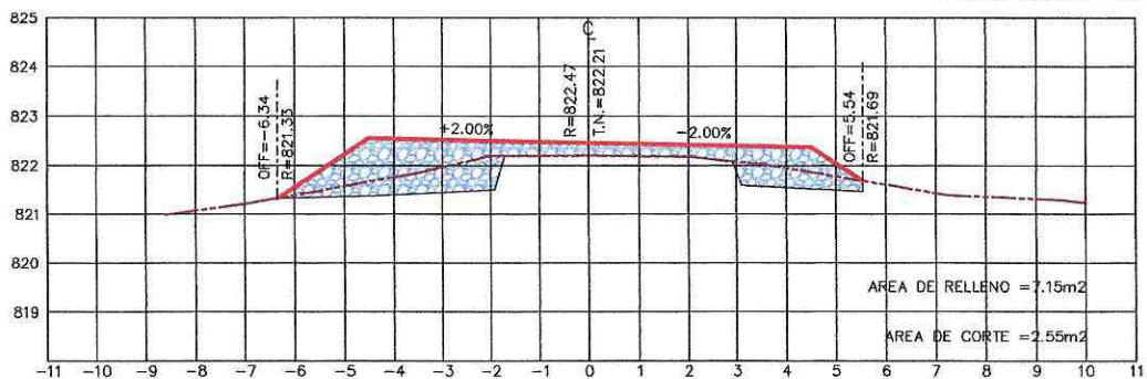
ESTACION 4+600.00 ESCALA HORIZONTAL 1 : 100 ESCALA VERTICAL 1 : 100
