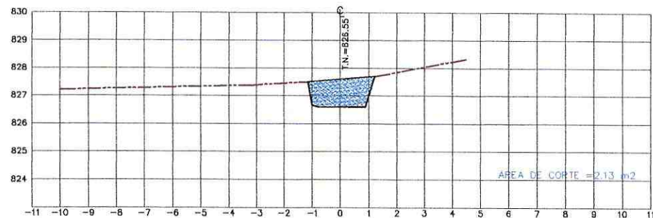
ESTACION 3+047.00 - Lado Izquierdo ESCALA HORIZONTAL 1 : 100 ESCALA VERTICAL 1 : 100
