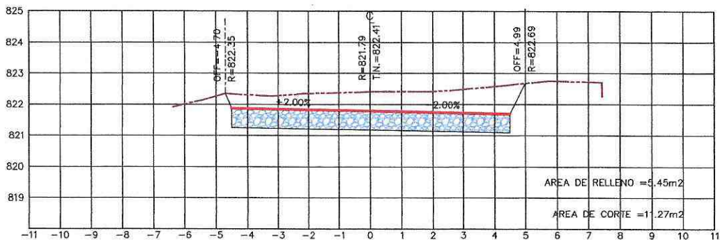
ESTACION 4+560.00 ESCALA HORIZONTAL 1 : 100 ESCALA VERTICAL 1 : 100
