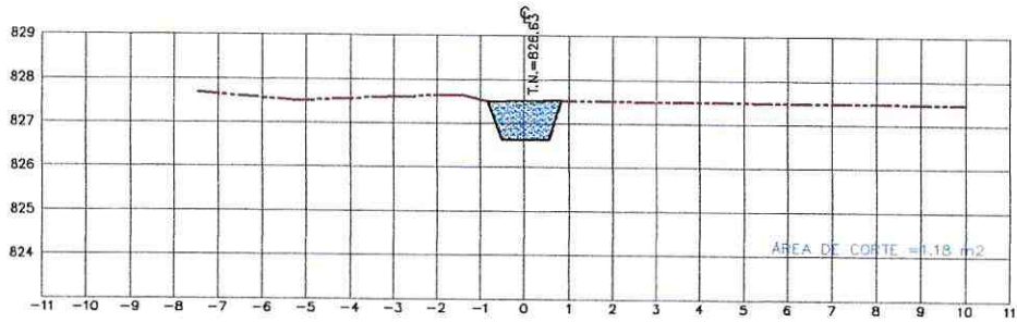
ESTACION 2+907.00 - Lado Derecho ESCALA HORIZONTAL 1 : 100 ESCALA VERTICAL 1 : 100
