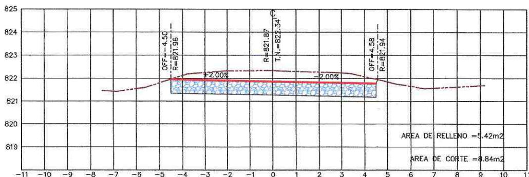
ESTACION 4+580.00 ESCALA HORIZONTAL 1 : 100 ESCALA VERTICAL 1 : 100
