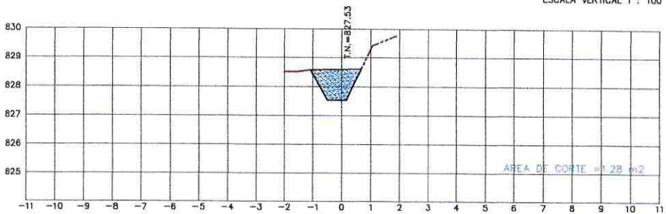
ESTACION 3+047.00 - Lado Derecho ESCALA HORIZONTAL 1 : 100 ESCALA VERTICAL 1 : 100
