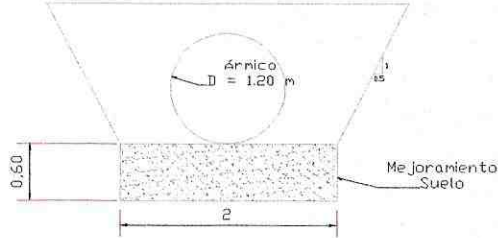
Sección Exc. y Relleno (Tub. D=1.20 m)
