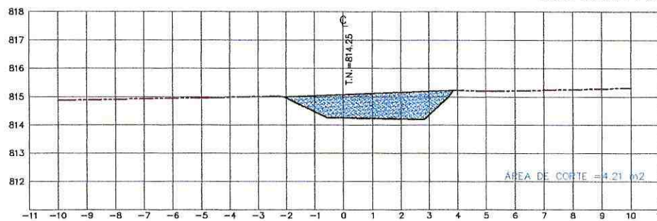
ESTACION 0+474.00 - Lado Izquierdo ESCALA HORIZONTAL 1 : 100 ESCALA VERTICAL 1 : 100
