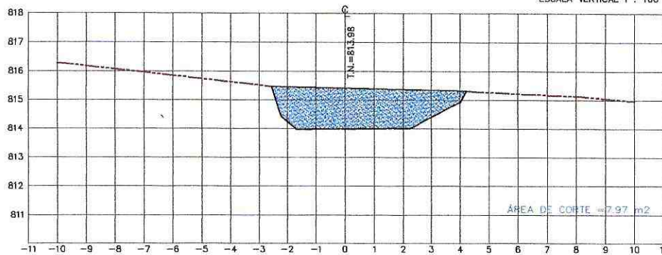
ESTACION 0+474.00 - Lado Derecho ESCALA HORIZONTAL 1 : 100 ESCALA VERTICAL 1 : 100
