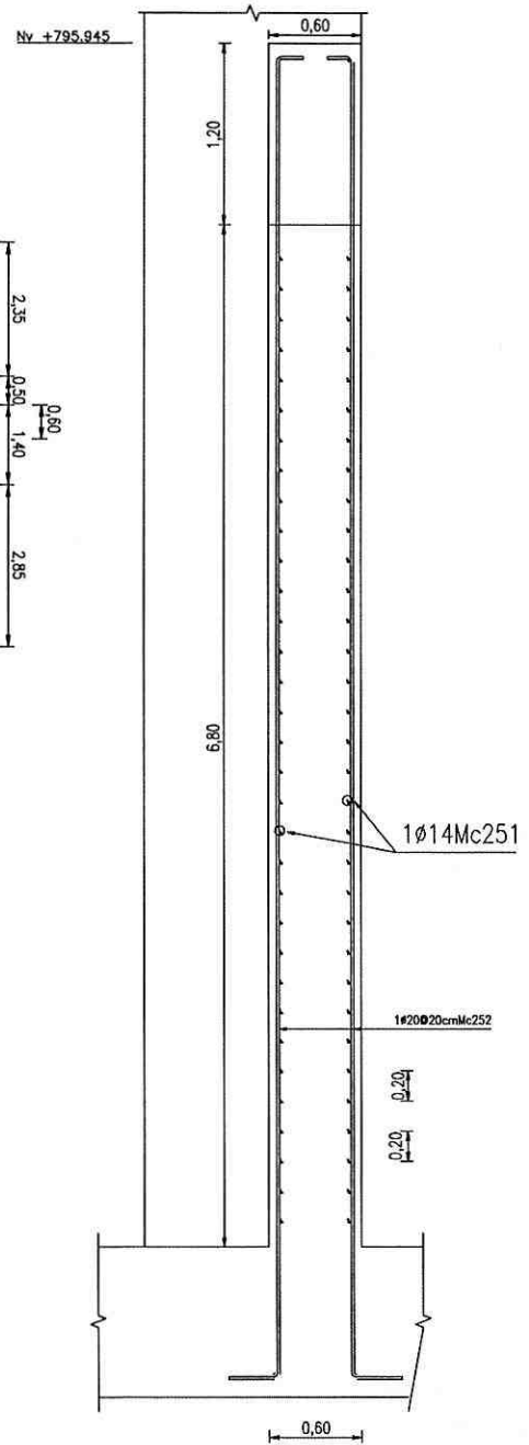
CORTE LATERAL DE MURO FRONTAL
