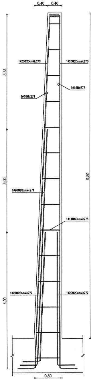
VISTA LATERAL MUROS DE ALA
