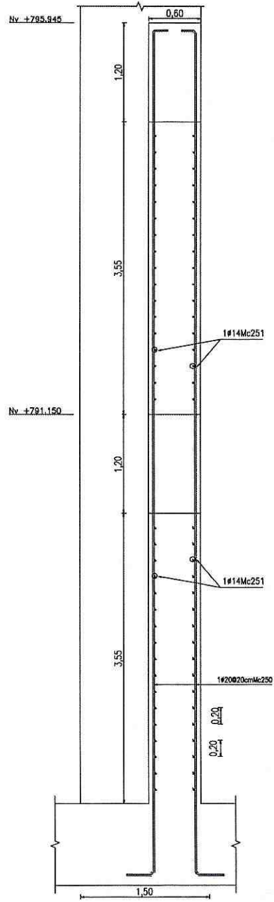
CORTE LATERAL MURO FRONTAL
