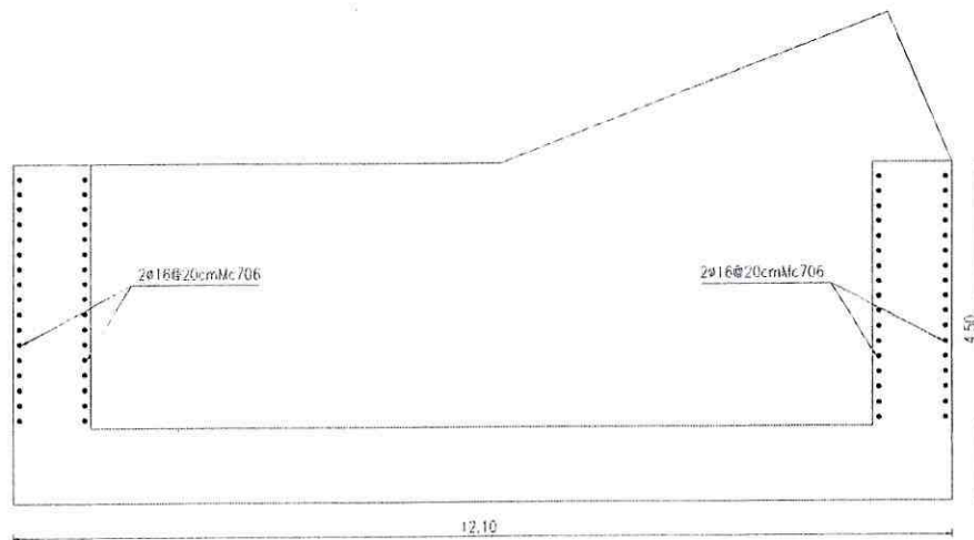
DETALLE DE ARMADO DE CAJON DE ANLAJE (CORTE A-A)
