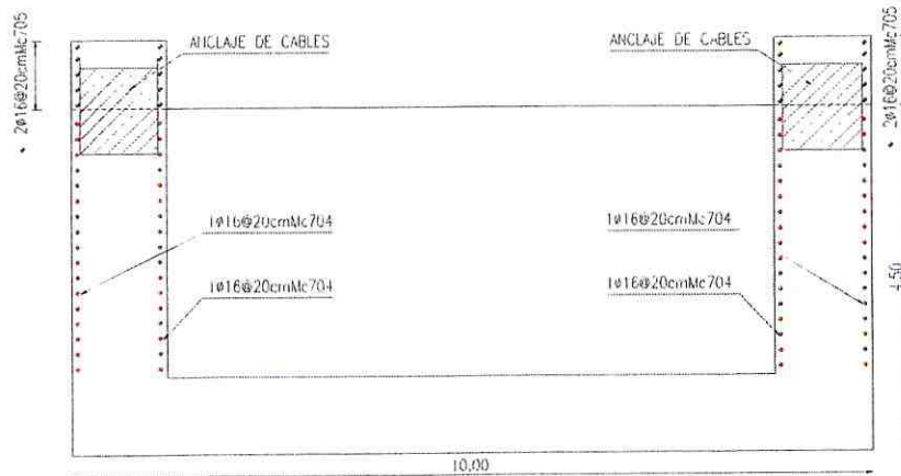
DETALLE DE ARMADO DE CAJON DE ANLAJE (CORTE B-B)
